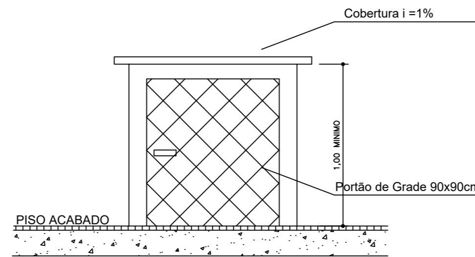
DETALHE DA CABINE DE INSTALAÇÃO DE GÁS COMBUSTIVEL /IN 08/DAT/CBMSC Escala: 1/25
