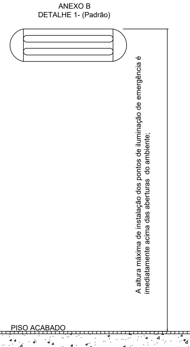
DETALHE DO SISTEMA DE ILUMINAÇÃO DE EMERGÊNCIA /IN 011/DAT/CBMSC Escala: 1/25
