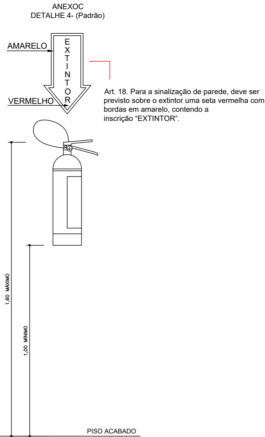
DETALHE DO SISTEMA PREVENTIVO POR EXTINTORES /IN 006/DAT/CBMSC Escala: 1/25
